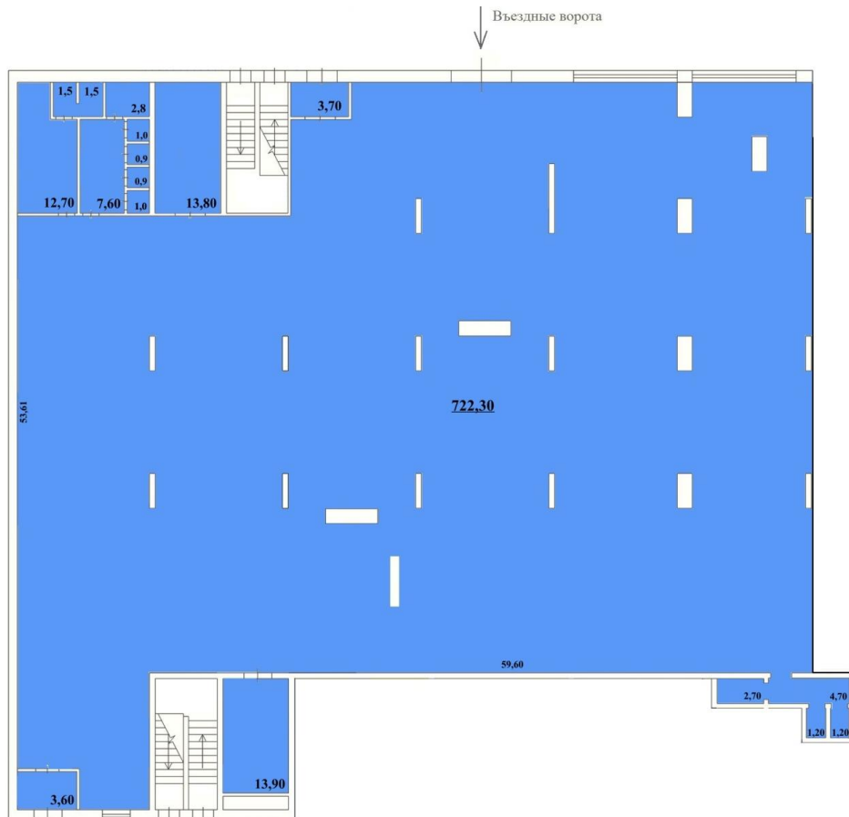
План помещения 788,60 кв.м.
